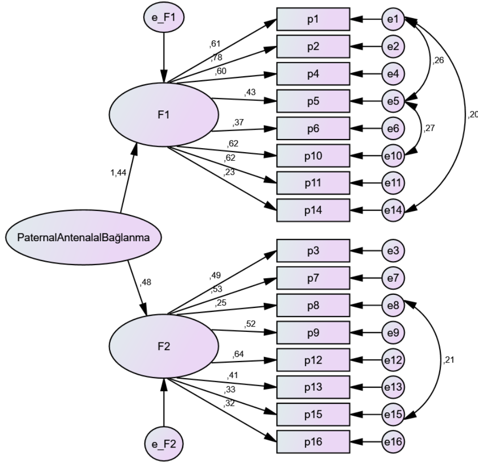
Şekil 1: Paternal Antenatal Bağlanma Ölçeğinin İkincil Düzey Çok Faktörlü Doğrulamalı Faktör Analizine İlişkin Yapısal Eşitlik Modeli
